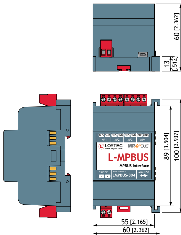
DIM051 LMPBUS-804
