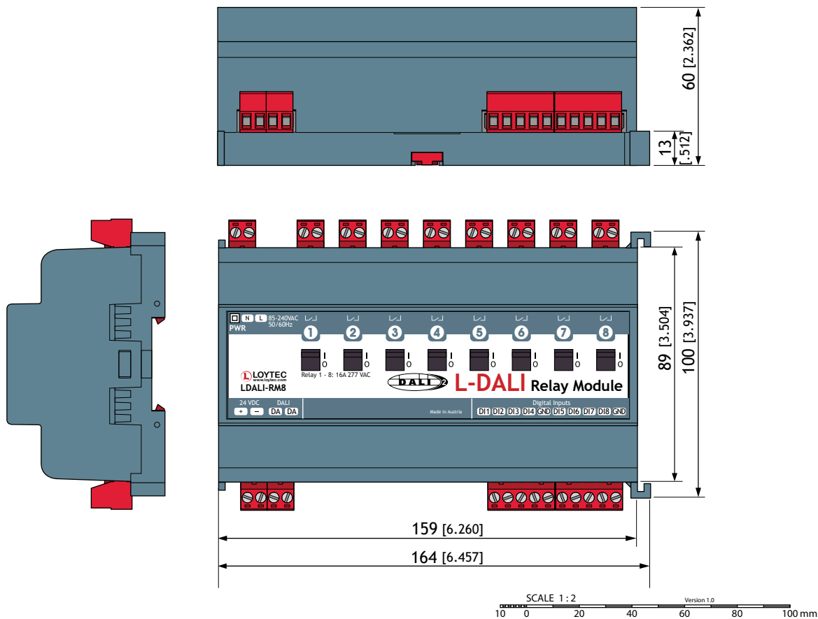
DIM064 LDALI-RM8
