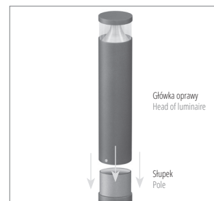
Główna oprawa i słup - przykład montażu Head and pole - example of mounting
