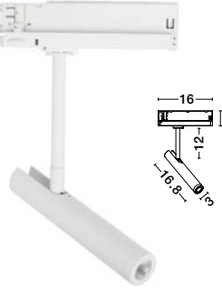
WANG - 9123132 12W · 3000K
