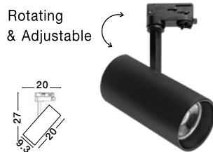
HERM - 7770410 · 30W · 3000K 8770413 · 30W · 4000K
