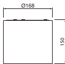
Xon-LED-25-1 Xon-LED-36-1
